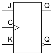
J-K Flip-flop
